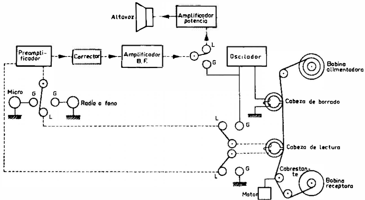
Esquema del principio de lectura en un magnetófono
