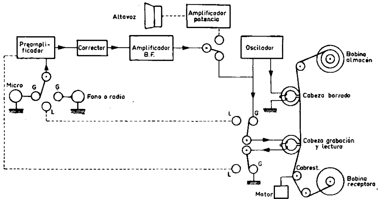
Esquema del principio de funcionamiento de la grabación magnetofónica
