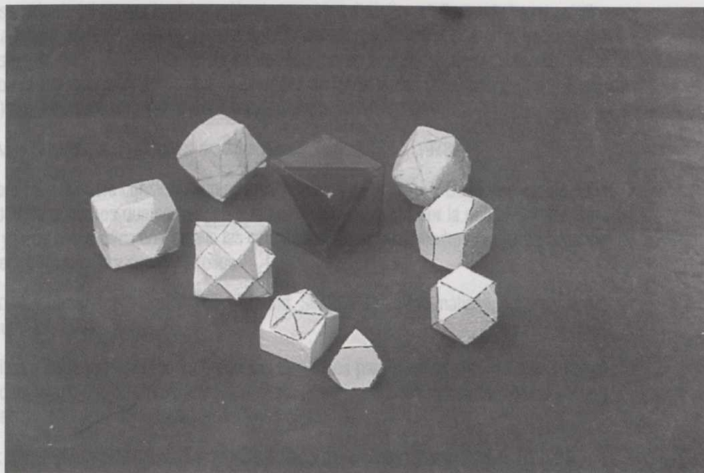
Foto 6. Truncamiento de Poliedros
