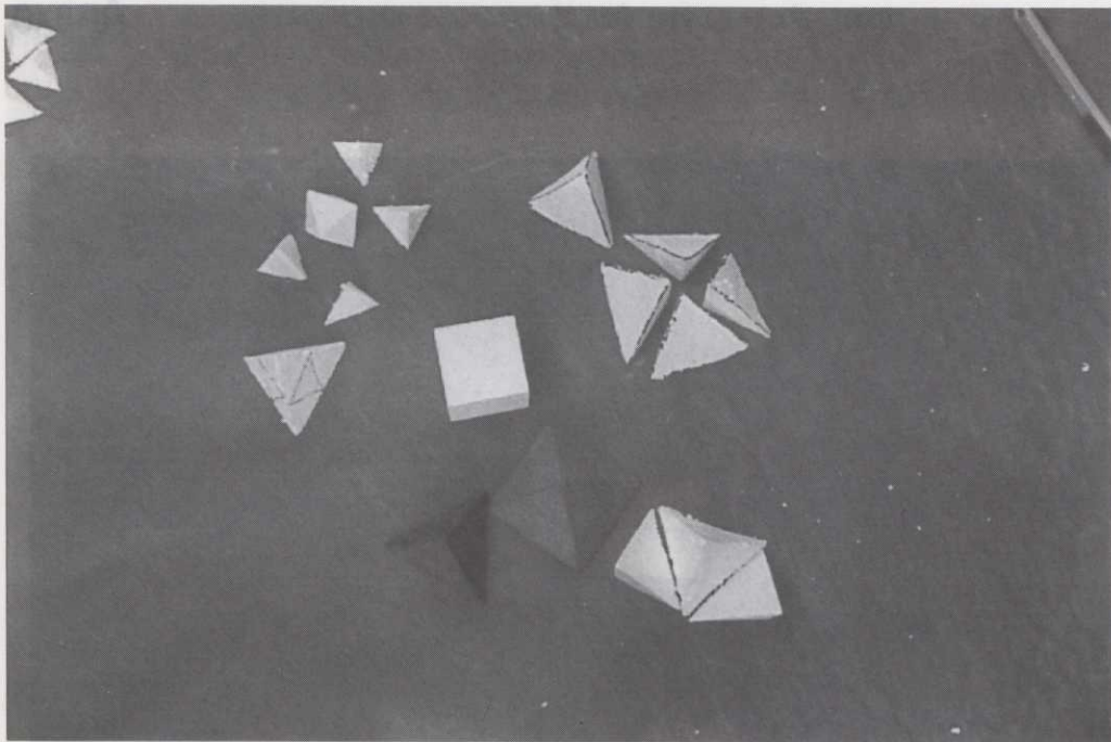
Foto 3. 1 \text{ cubo} = 1 \text{ tetraedro} + 1/2 \text{ octaedro} 1 \text{ tetraedro} = 1 \text{ octaedro} + 4 \text{ tetraedros}
