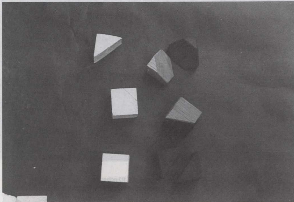
Foto 1. Descomposición de un cubo. Secciones planas
