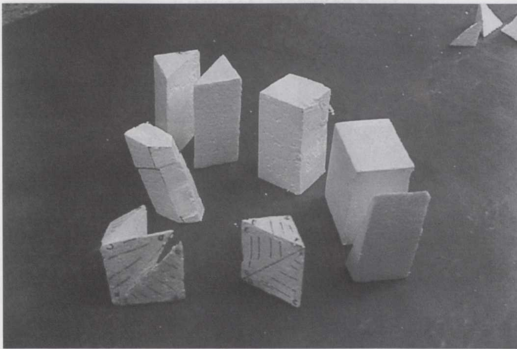
Foto 4. Descomposición de prismas. Equivalencias
