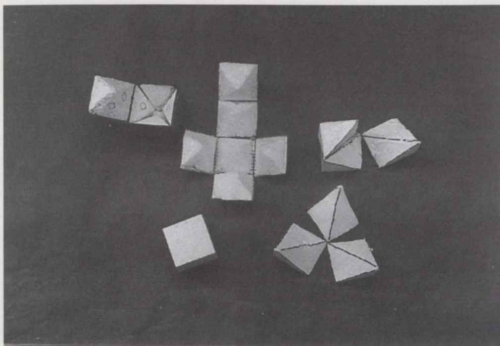
Foto 2. 1 cubo = 3 pirámides equivalentes 1 cubo = 6 pirámides equivalentes
