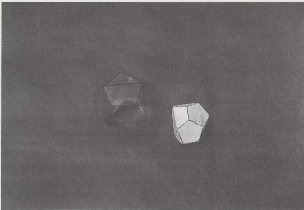
Foto 5. El cubo en el dodecaedro
