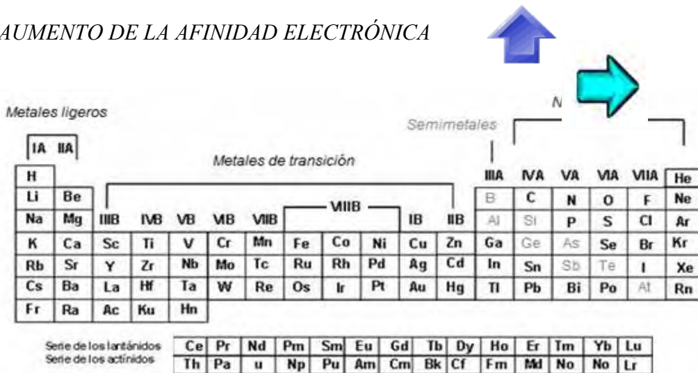
Fig. 8. Aumento general de la afinidad electrónica en la tabla periódica
