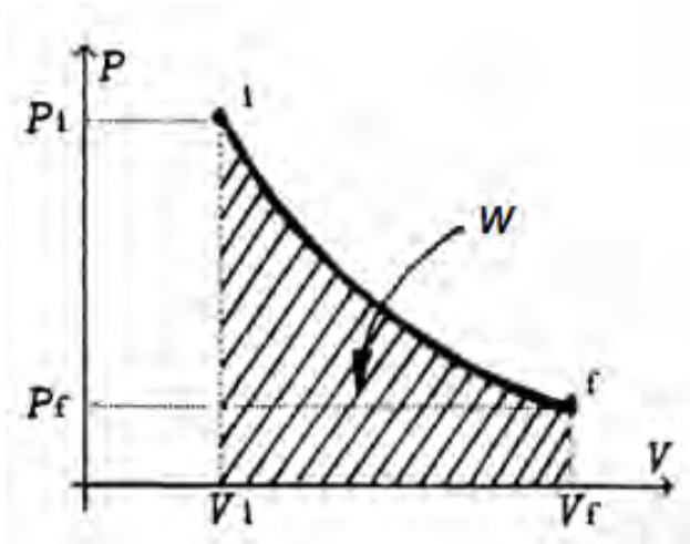
Fig. 1. Representación de los estados de un gas como una curva, en un diagrama P - V
