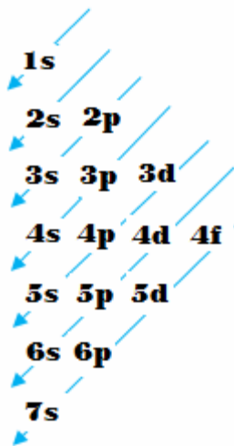
Fig 4. Diagrama de orden de llenado de orbitales atómicos
