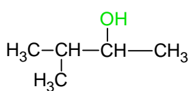
alcohol secundario
