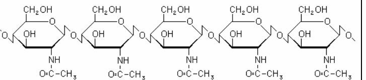
Quitina N-acetil-D-glucopiranosil \beta (1→4)
