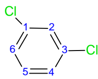
meta-diclorobenceno
