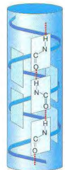
Hélice alfa
