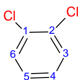
orto-diclorobenceno
