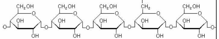
Celulosa D-glucopiranosil \beta (1→4)
