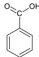
Ácido benzoico
