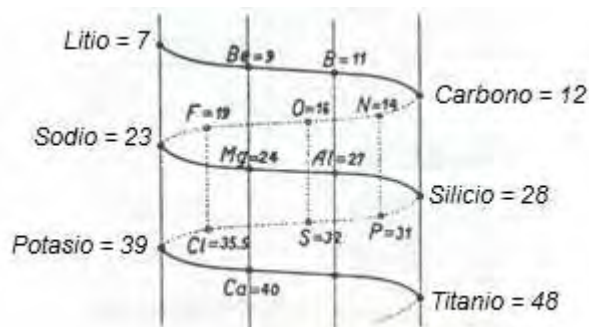
Fig. 2. Diagrama de Chancourtois
