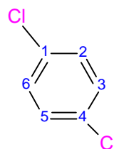
para-diclorobenceno
