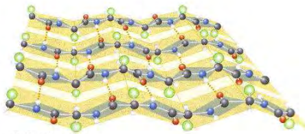
Lámina beta
