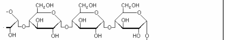
Amilopectina o Glucógeno D-glucopiranosil \alpha (1→4), \alpha (1→6)
