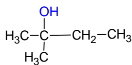
alcohol terciario
