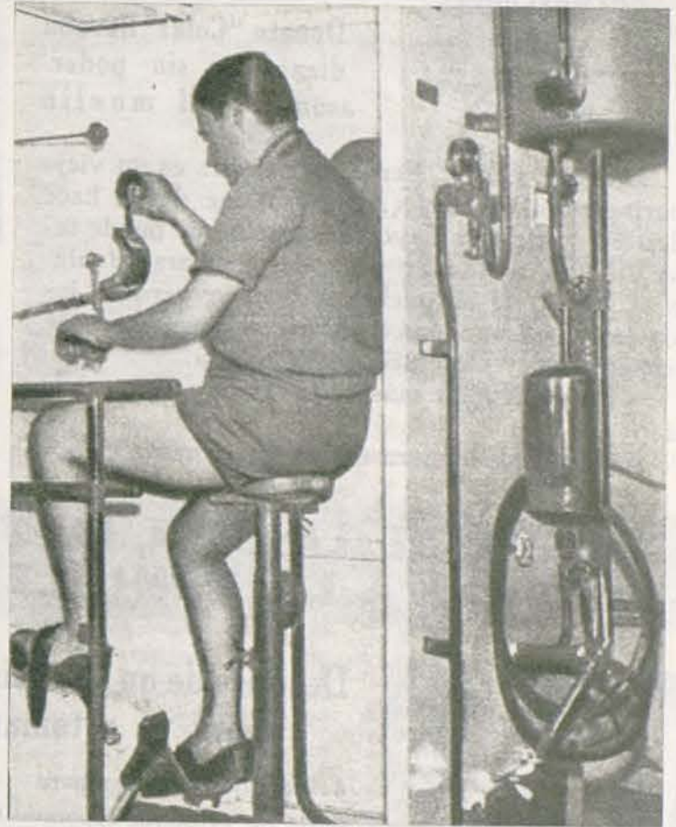
Joaquín Constantino Garay, con el aparato de su invención para la rehabilitación de enfermos reumáticos.
